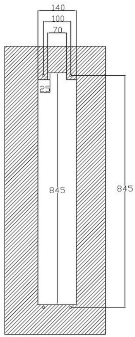
Wymiary otworu montażowego IRGLASSPA
